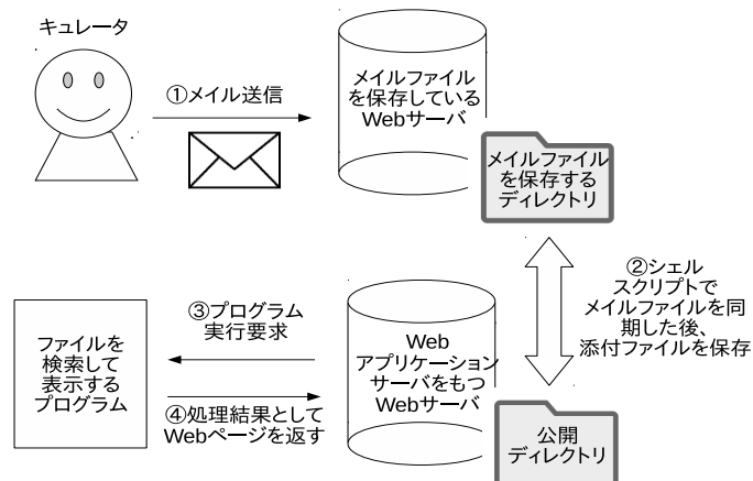
図 4.7: MTA を利用したプログラムの実行の流れ
