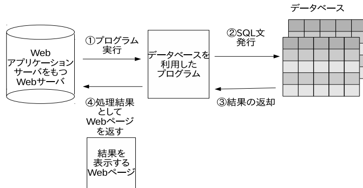
図 4.6: データベースを利用したプログラムの実行の流れ
