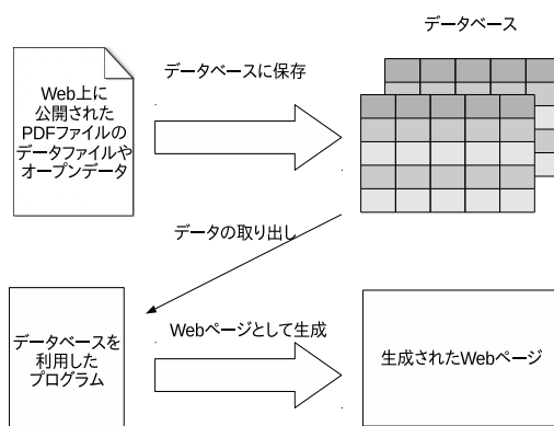
図 2.2: データベースを利用したプログラムの概観
