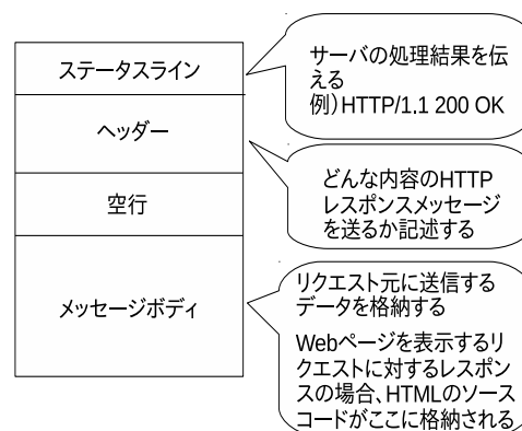
図 4.2: HTTP レスポンスの内容
