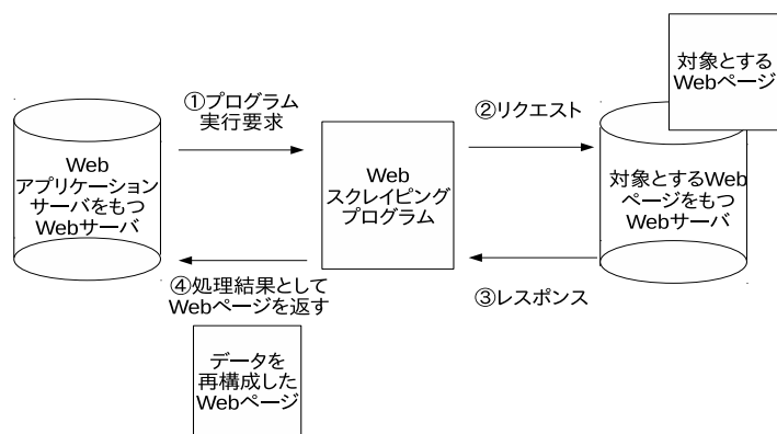
図 4.5: Web スクレイピングプログラムの実行の流れ
