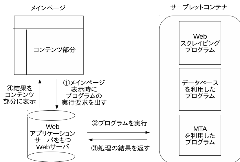
図 4.4: システムの実行の流れ
